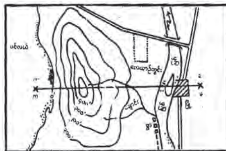
ပုံ (၂) ကွန်တိုမျဉ်းများပေါ် အမြင့်ပေများမှတ်သားပုံ
